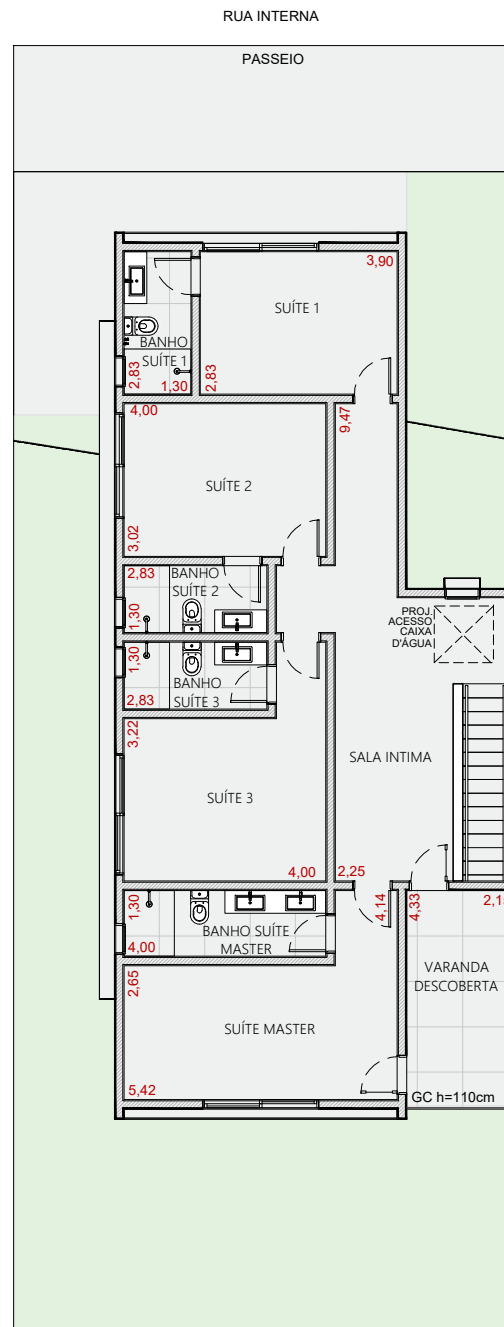
PLANTA SUPERIOR ESC.: 1:150
