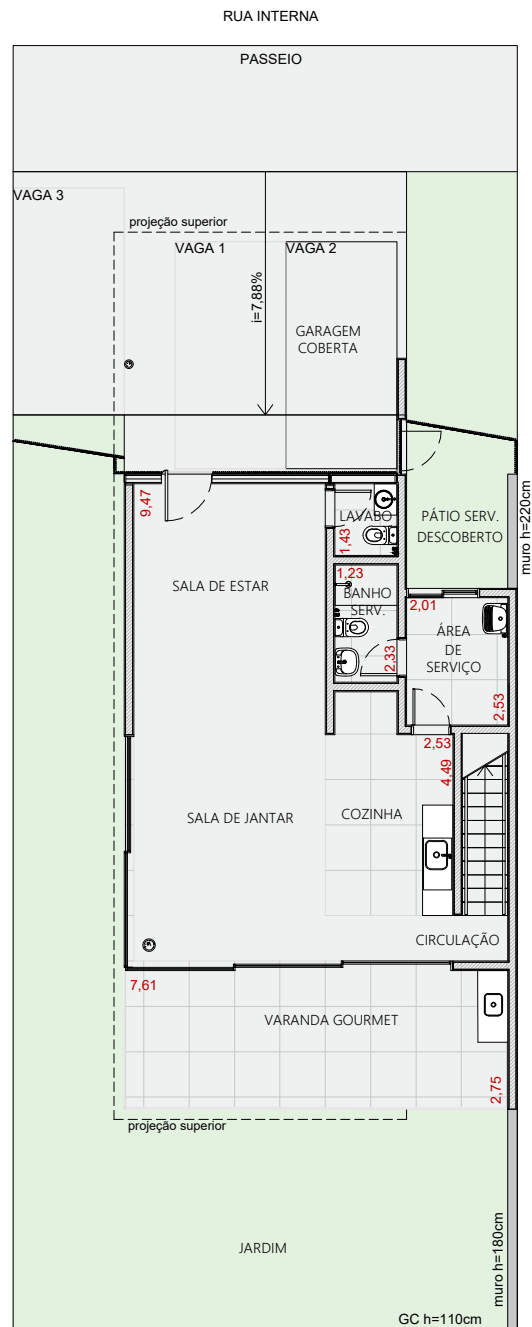
PLANTA TÉRREO ESC.: 1:150
